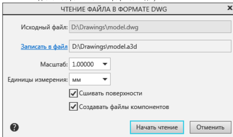
Диалог настройки чтения в модель
