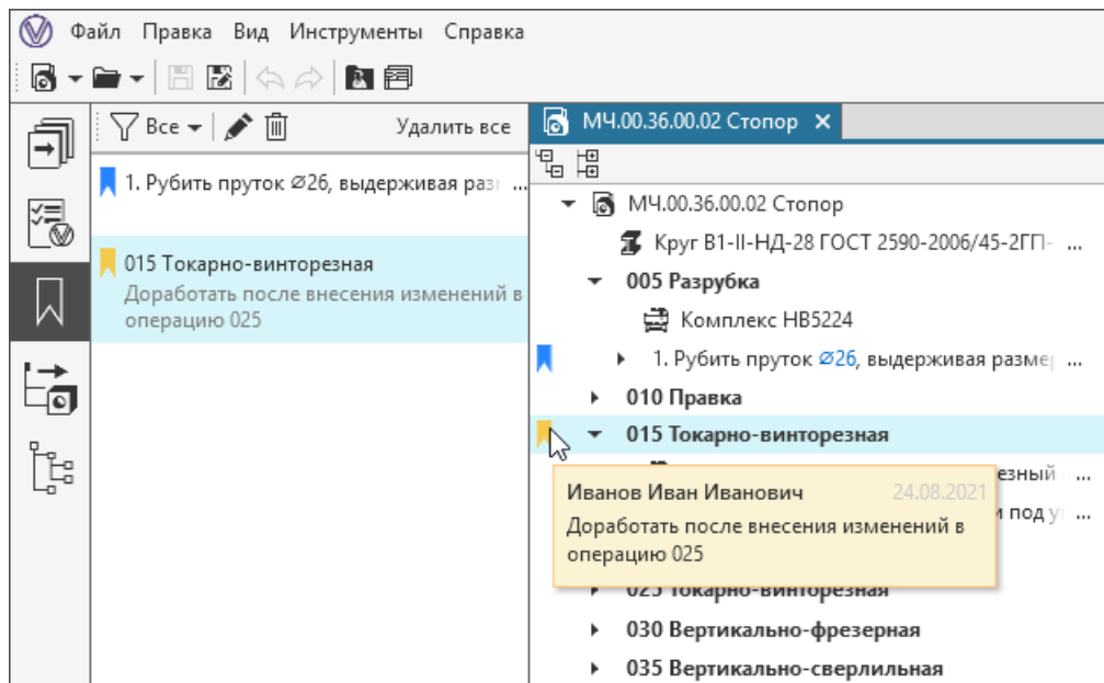
Отображение панели управления закладками
