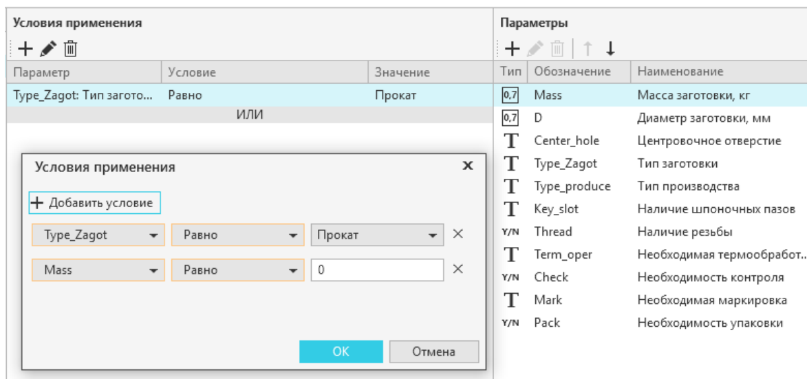
Добавление условий применения объектов
