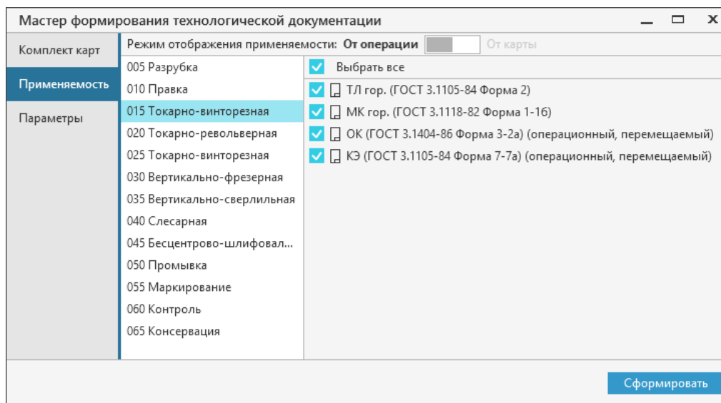
Настройка применяемости карт в режиме отображения От операции
