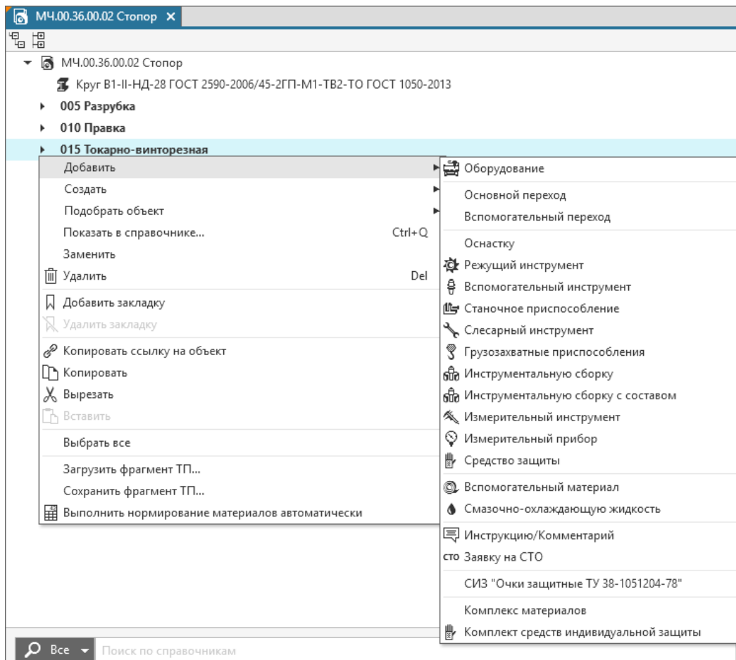
Контекстное меню объекта Операция
