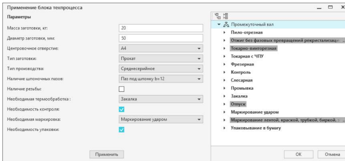
Управление параметрами условий применения блока техпроцесса
