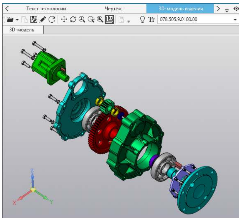
Применение команды Разнести к 3D-модели сборки
