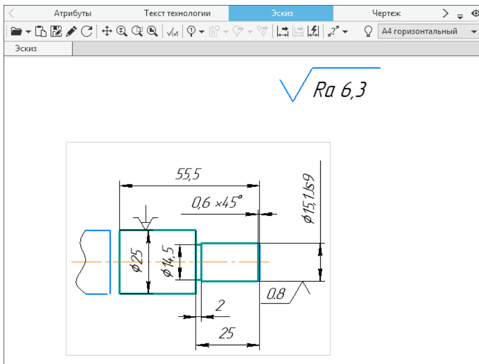
Вкладка Эскиз
