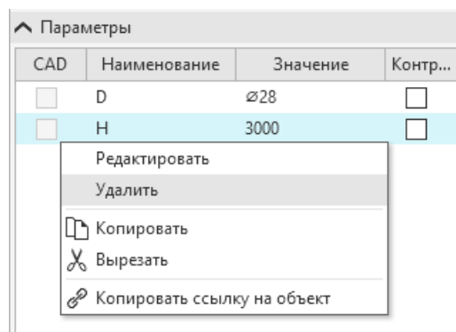
Удаление параметра
