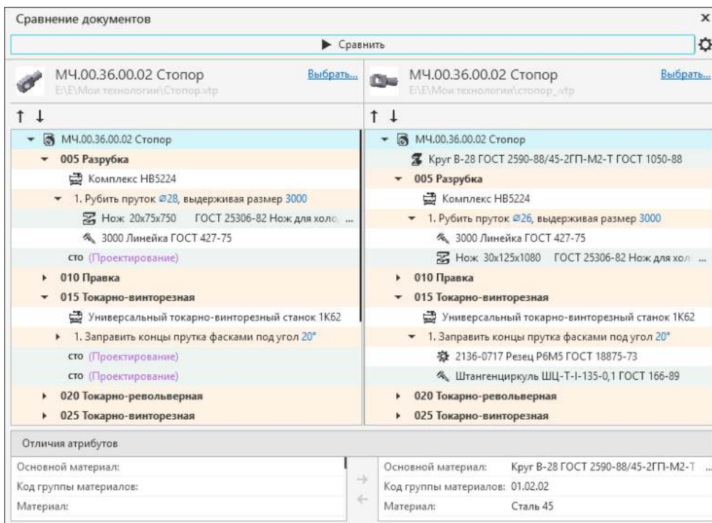
Результат сравнения техпроцессов
