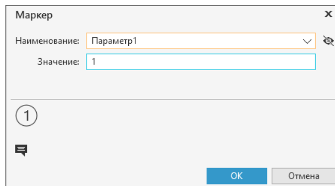
Диалог Маркер
