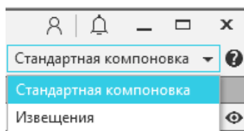
Переключатель компоновки
