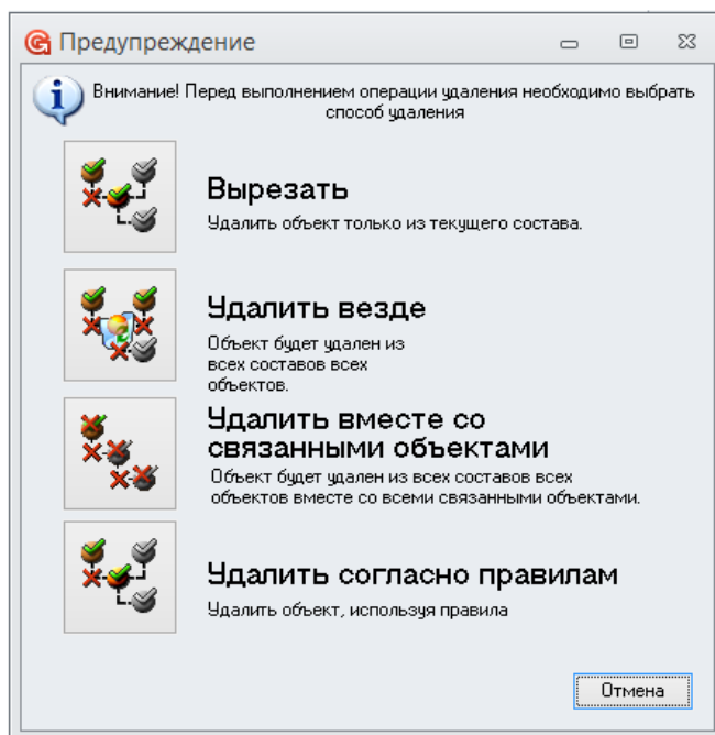
Рисунок 22: Окно "Предупреждение"
