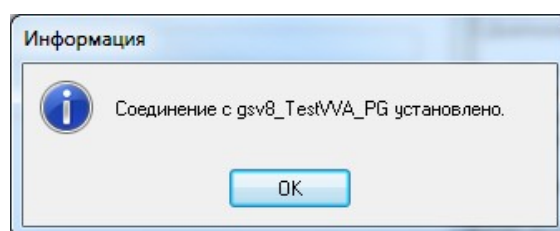
Рисунок 252: Пример сообщения
