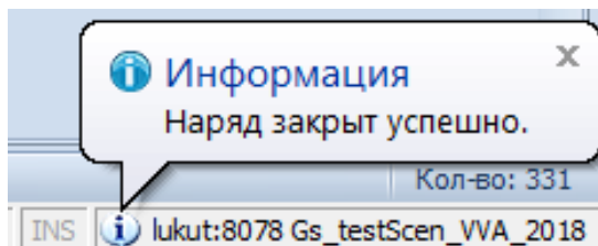
Рисунок 152. Пример сообщения
