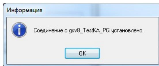
Рисунок 250: Пример сообщения
