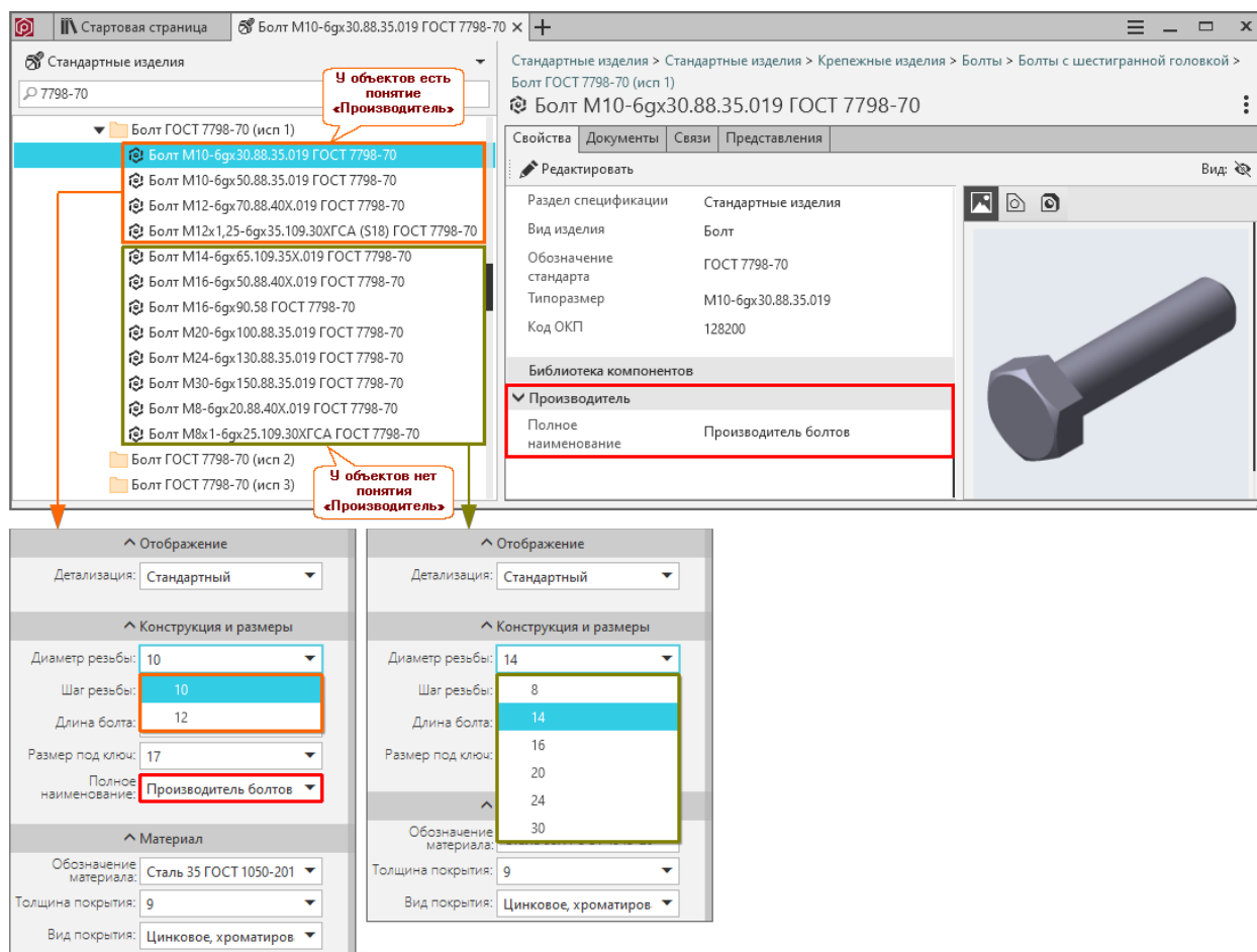
Панели параметров в КОМПАС-3D при вставке объектов справочника
